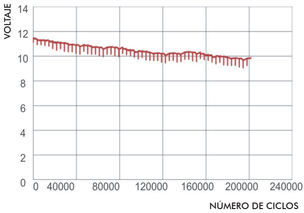
CURVA DE VIDA DE PARADA EN RALENTÍ
