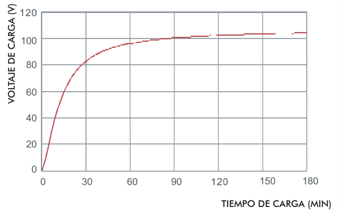
CURVA DE RENDIMIENTO DE CARGA RÁPIDA
