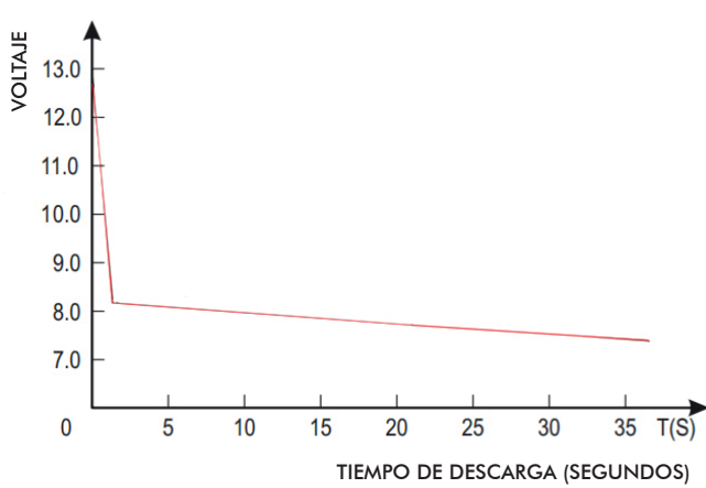
CURVA DE AUTODESCARGA A -18°C (0°F)
